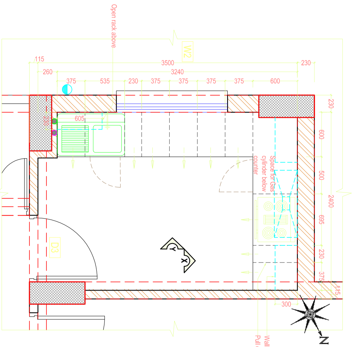
PLAN 'P1-P1'
